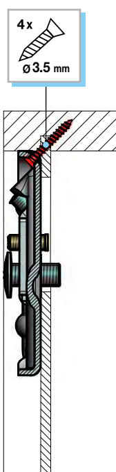
SEZ. B-B
